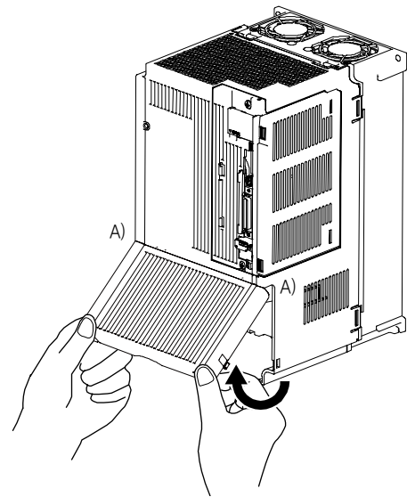
2) ㉠을 지점으로 해, 끌어올리듯이 커버를 들어 올립니다.
