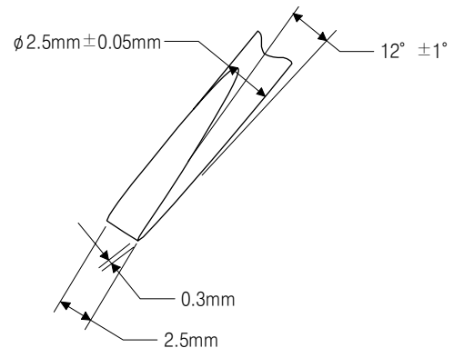
드라이버의 형태 \phi 2.5\text{mm}
