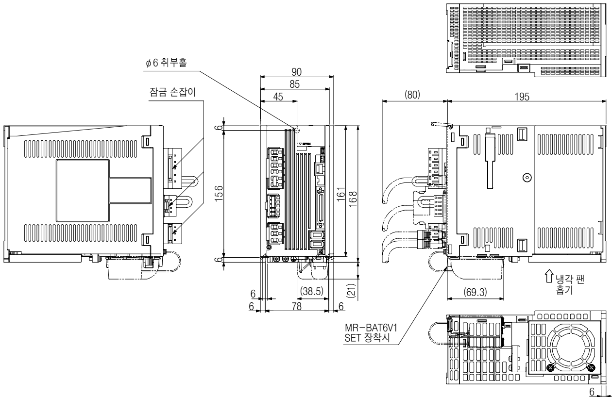
(d) MR-J4-200A(-RJ)
