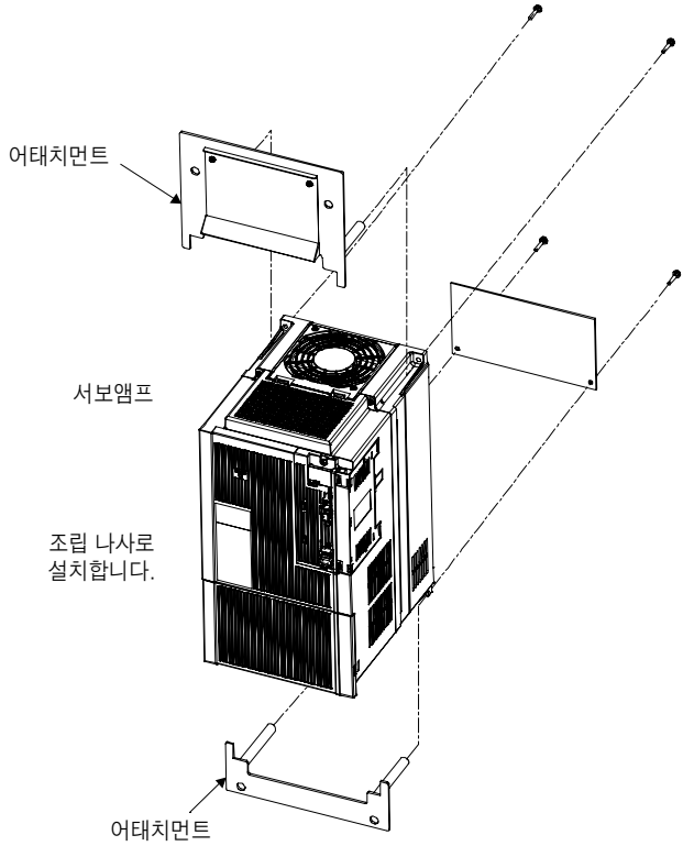
a. 냉각핀 외부 노출 어태치먼트의 조립
