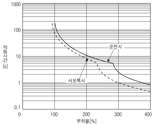
b. LM-U2시리즈
