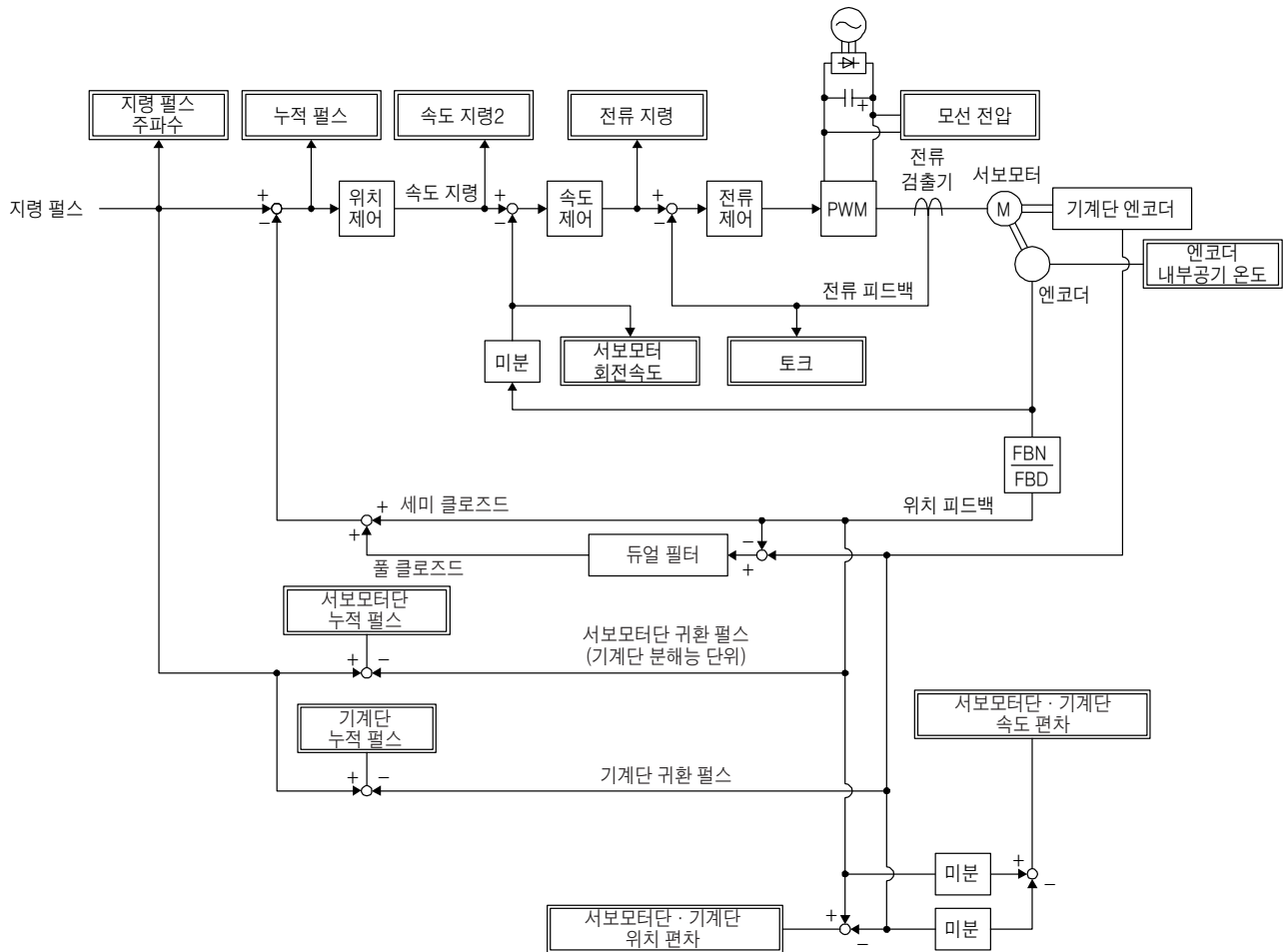
(b) 폴 클로즈드 제어
