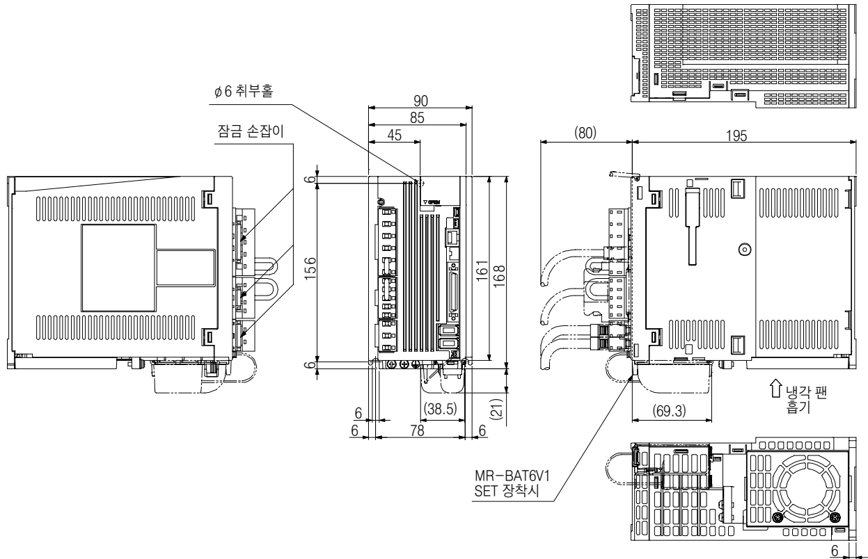
(b) MR-J4-200A4(-RJ)
