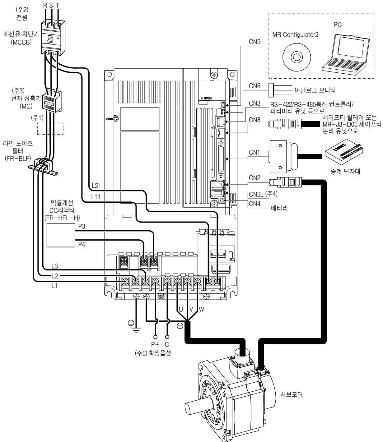
(d) MR-J4-700A4(-RJ)
