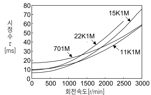
HG-JR 1500r/min 시리즈
