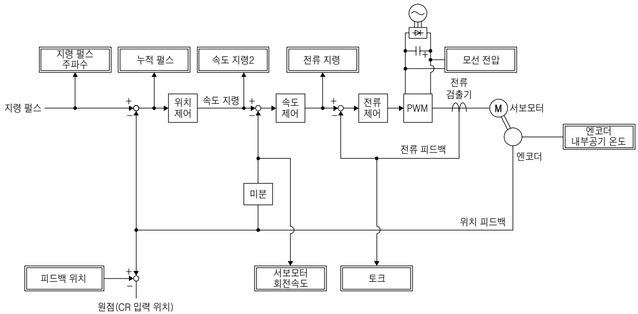
(a) 세미 클로즈드 제어
